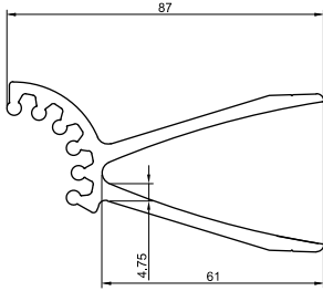
منقاری لوور End cap louver az-7011 1950gr/m
