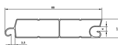
تیغه ۶۰ blade 60 az-600 340gr/m
