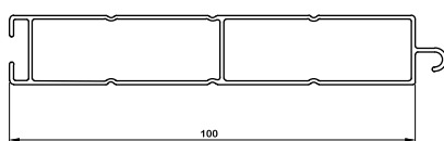
ریل بغل side rail az-102 940gr/m
