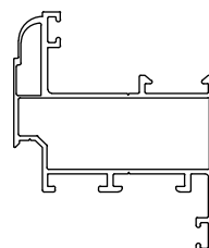
بازشو لولایی پنجره opening hinged window az-5200 1000gr/m
