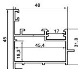
وسطی دولنگه لولایی hinged middle double leaf az-5249 850gr/m
