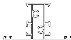
سپری لولایی hinged Tprofile
