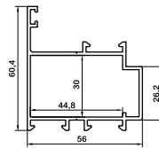
چهارچوب درب لولایی double wall frame az-5251 1050gr/m
