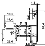
وسطی دولنگه لولایی enter hinged double leaf az-6249/tr 1070gr/m
