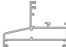
کتیبه لولایی hinged coping az-1253 820gr/m
