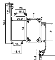
بازشو درب لولایی opening hinged door az-6201/tr 1460gr/m
