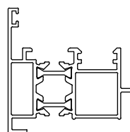
وسطی دولنگه لولایی enter hinged double leaf
