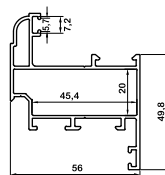
بازشو لولایی پنجره opening hinged window az-5200 1000gr/m
