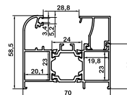
چهارچوب پنجره لولایی Window hinged frame az-6250/tr 1100gr/m
