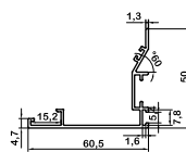
رابط اسپانیولت espagnolette joint az-6015/tr 200gr/m
