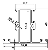
ریل توری کشویی sliding net rail az-5508 340gr/m
