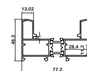
بازشو کشویی sliding opening az-6202/tr 1700gr/m
