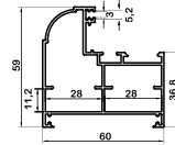
چهارچوب درب لولایی double wall frame az-1251 1150gr/m
