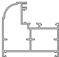
چهارچوب درب لولایی
