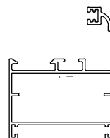
چهارچوب لولایی سبک Window hinged frame
