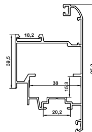
بیرون بازشو درب لولایی out side opening hinged door azL-1201/2 1150gr/m
