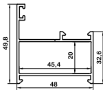
چهارچوب لولایی پنجره Window hinged frame az-5250 750gr/m
