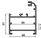
چهارچوب لولایی سبک light weight hinged frame az-1250 750gr/m
