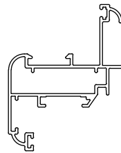
بازشو لولایی سبک Light weight opening az-1200 770gr/m
