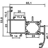
بازشو پنجره لولایی opening hinged window az-6200/tr 1200gr/m
