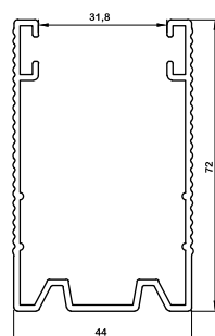
ریل بغل side rail az-101 960gr/m
