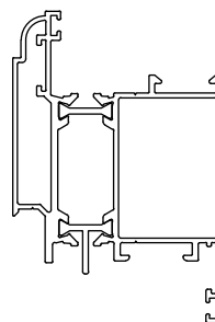
بازشو درب لولایی opening hinged door
