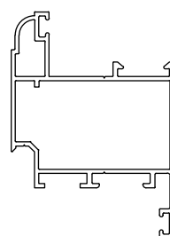
بازشودرپ لولایی opening hinged door az-5201 1150gr/m
