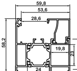
چهارچوب پنجره لولایی Window hinged frame az-6250/tr 1100gr/m
