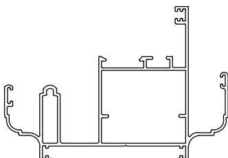
چهارچوب تک ریل کشویی mono rail sliding frame
