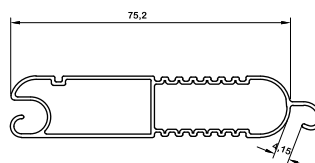
ریل بغل side rail az-101 960gr/m
