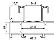
سپری لولایی hinged T profile az-5400 940gr/m
