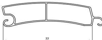
تیغه ۸۰ تخت لوکس blade 80 flat lux az-807 580gr/m
