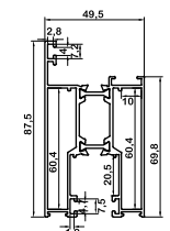
وسطی چهارلنگه middle four casement az-6014/tr 600gr/m
