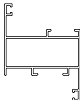
بازشو پنجره لولایی opening hinged window
