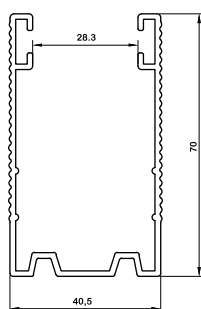
ریل بغل side rail az-102 940gr/m
