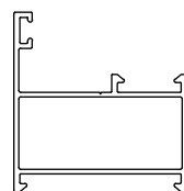
چهار چوب لولایی پنجره Window hinged frame az-5250 750gr/m
