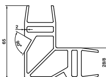
قید وسط درب door middle frame az-5351 1900gr/m
