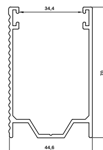
تیغه ۶۰ blade 60 az-103 1000gr/m
