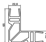
سپری لولایی hinged Tprofile az-6400/tr 1250gr/m
