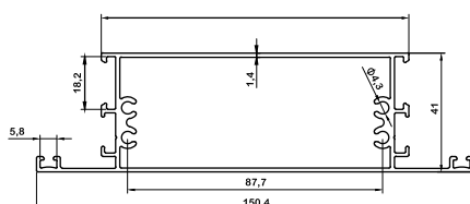
سپری بزرگ لولایی Sliding large T profile azL-1401/1 1720gr/m
