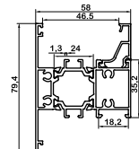
سپری لولایی hinged Tprofile az-6400/tr 1250gr/m
