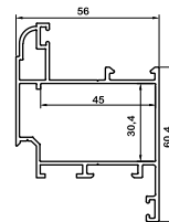
بازشودرب لولایی opening hinged door az-5201 1150gr/m
