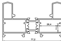
چهارچوب درب کشویی sliding double wall seal
