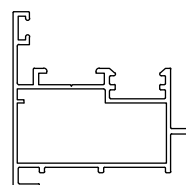
وسطی دولنگه لولایی sliding middle double leaf az-5249 850gr/m
