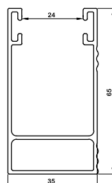
ریل بغل side rail az-104 860gr/m
